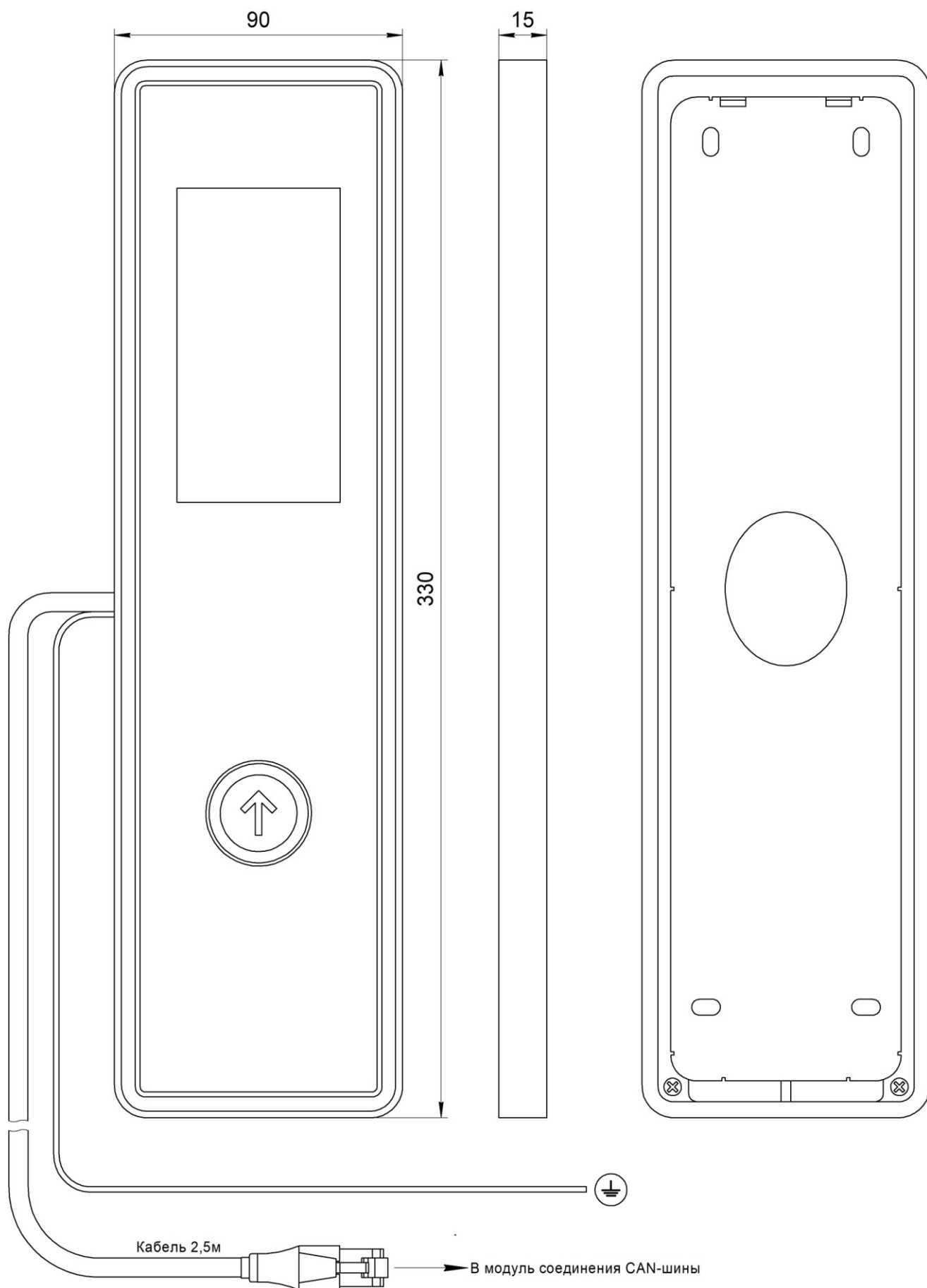
Рис.1 Внешний вид, габаритные и установочные размеры Вызывного поста ОБСИДИАН (жгут RJ45) НШЕК.468381.227
